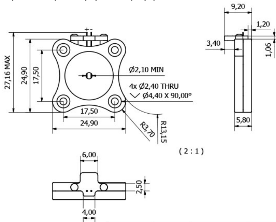
Чертеж 3 «Чертеж корпуса сенсора формальдегида»
