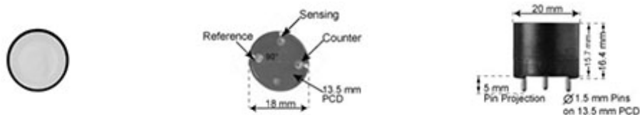
Чертеж 1 «Чертеж корпуса сенсора электрохимического»
