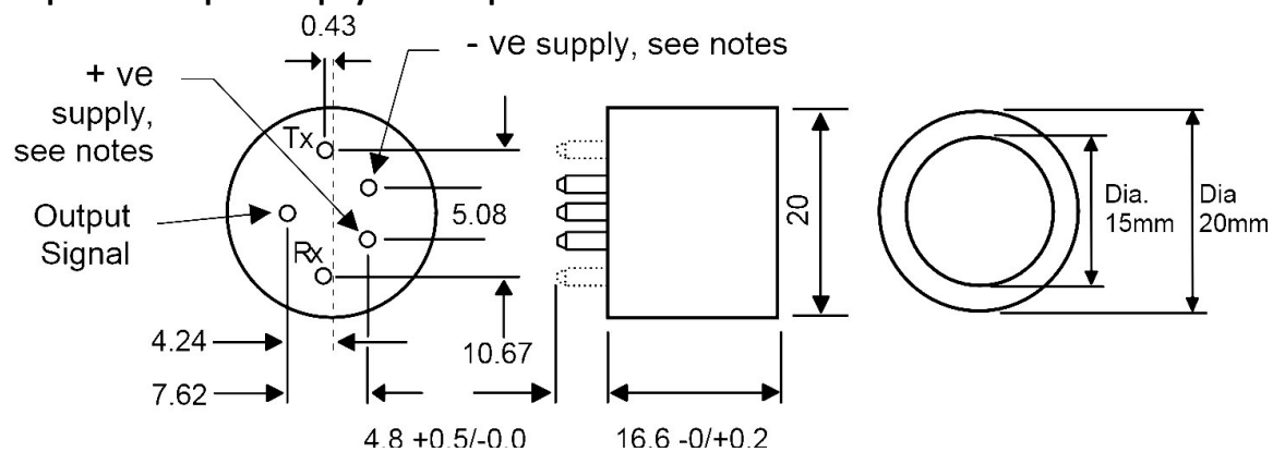
Чертеж 2 «Чертеж корпуса сенсора оптического»
