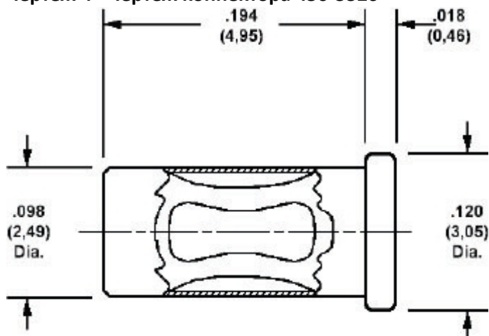
Чертеж 4 «Чертеж коннектора 450-3326»
